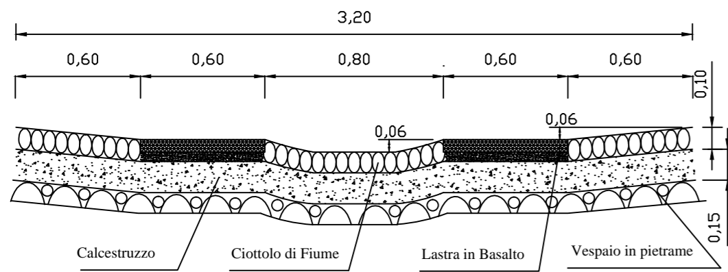
Sezione stradale Tipo Scala 1:10
